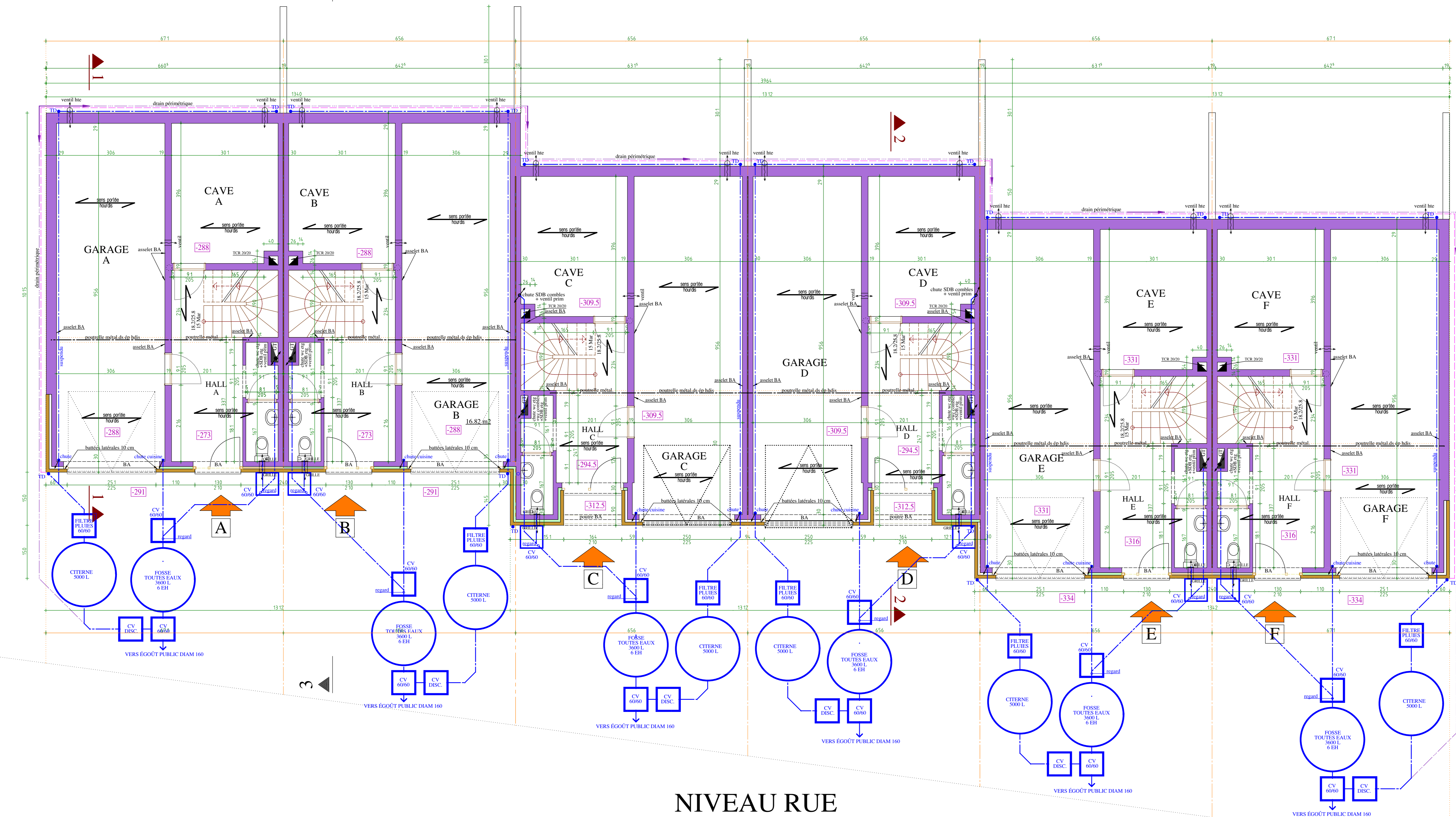
FAÇADE AVANT
